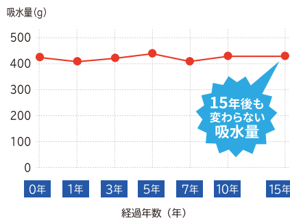
長期保存サンプル(7g)の 吸水量測定結果(生理食塩水吸水量)
